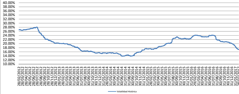
Gráfico de Volatilidad SX8E Index
